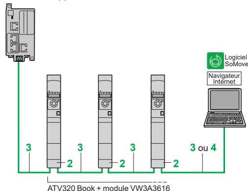
Exemple de raccordement sur réseau Ethernet/IP
