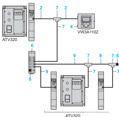
Exemple d'un raccordement multipoint
