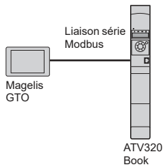
Exemple de configuration sur liaison série Modbus
