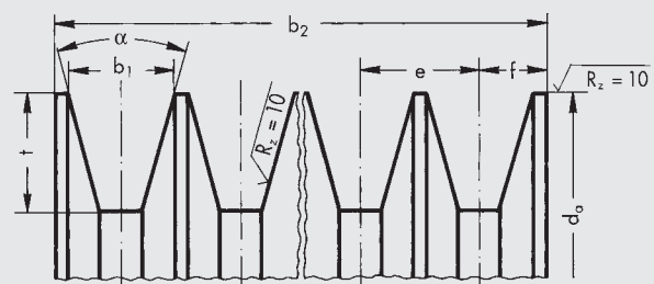
Poulie de mesure pour courroies jumelées
