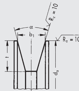
Poulie de mesure pour courroies trapézoïdales étroites de haute capacité norme américaine RMA/MPTA
