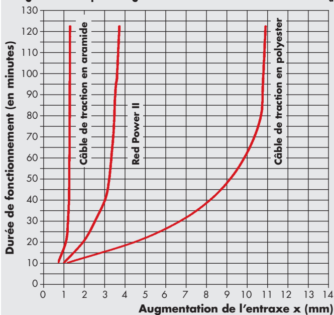
Banc d'essai - augmentation de l'entraxe [mm]
