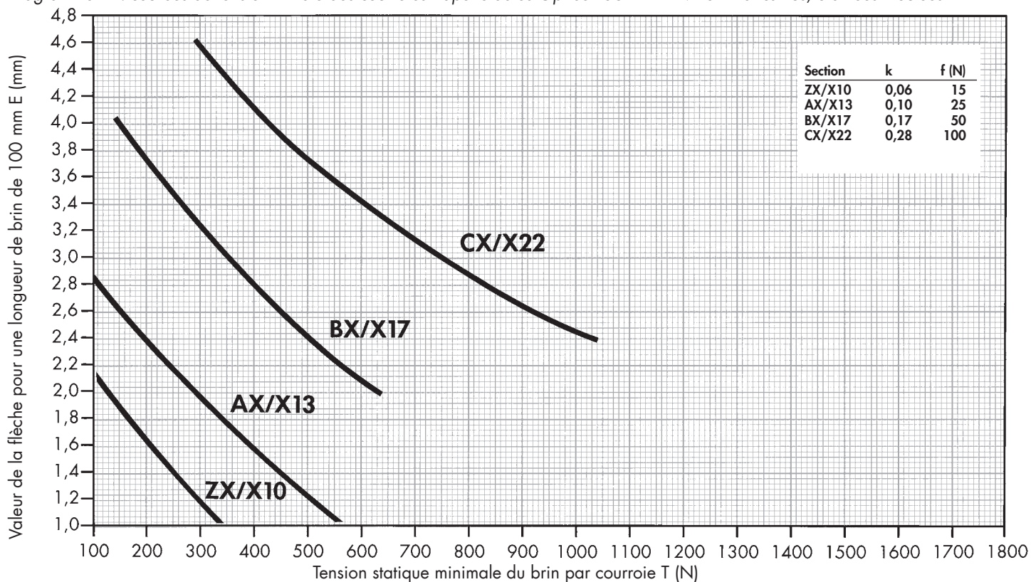
Diagramme 11: courbes de tension initiale des courroies trapézoïdales Optibelt SUPER TX M=S – flancs nus, crantées moulées
