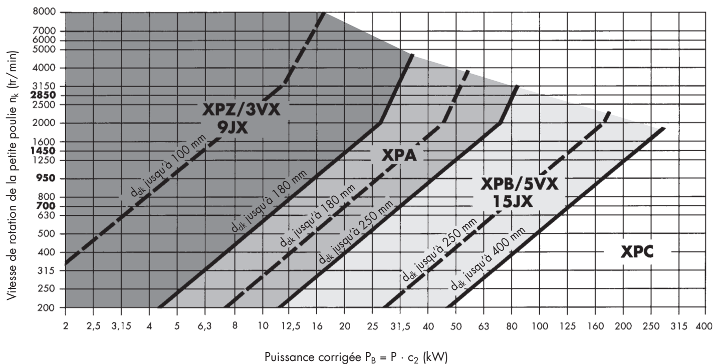
Diagramme 4: Courroies trapézoïdales étroites Optibelt Super X-POWER M=S
