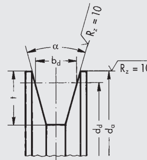
Poulie de mesure pour courroies trapézoïdales étroites de haute capacité DIN 7753 Partie 1 et courroies trapézoïdales classiques DIN 2215
