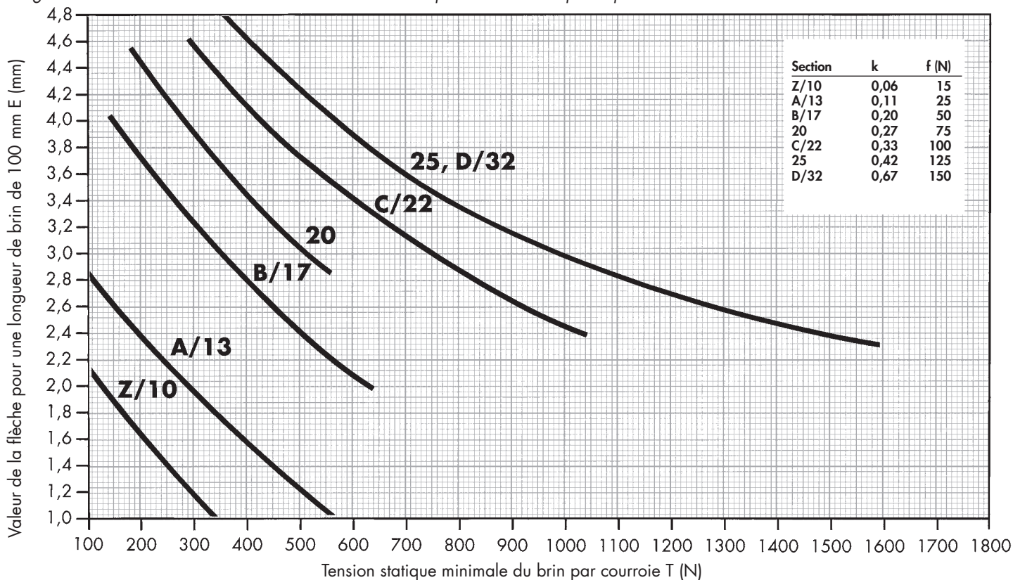
Diagramme 9: courbes de tension initiale des courroies trapézoïdales classiques Optibelt VB selon DIN 2215
