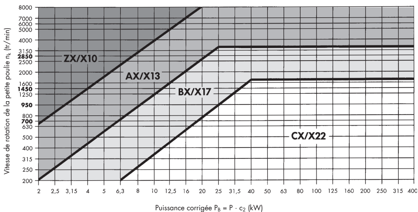
Diagramme 5: Courroies trapézoïdales Optibelt SUPER TX M=S
