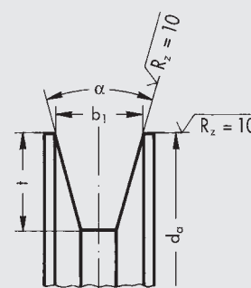
Poulie de mesure pour courroies hexagonales
