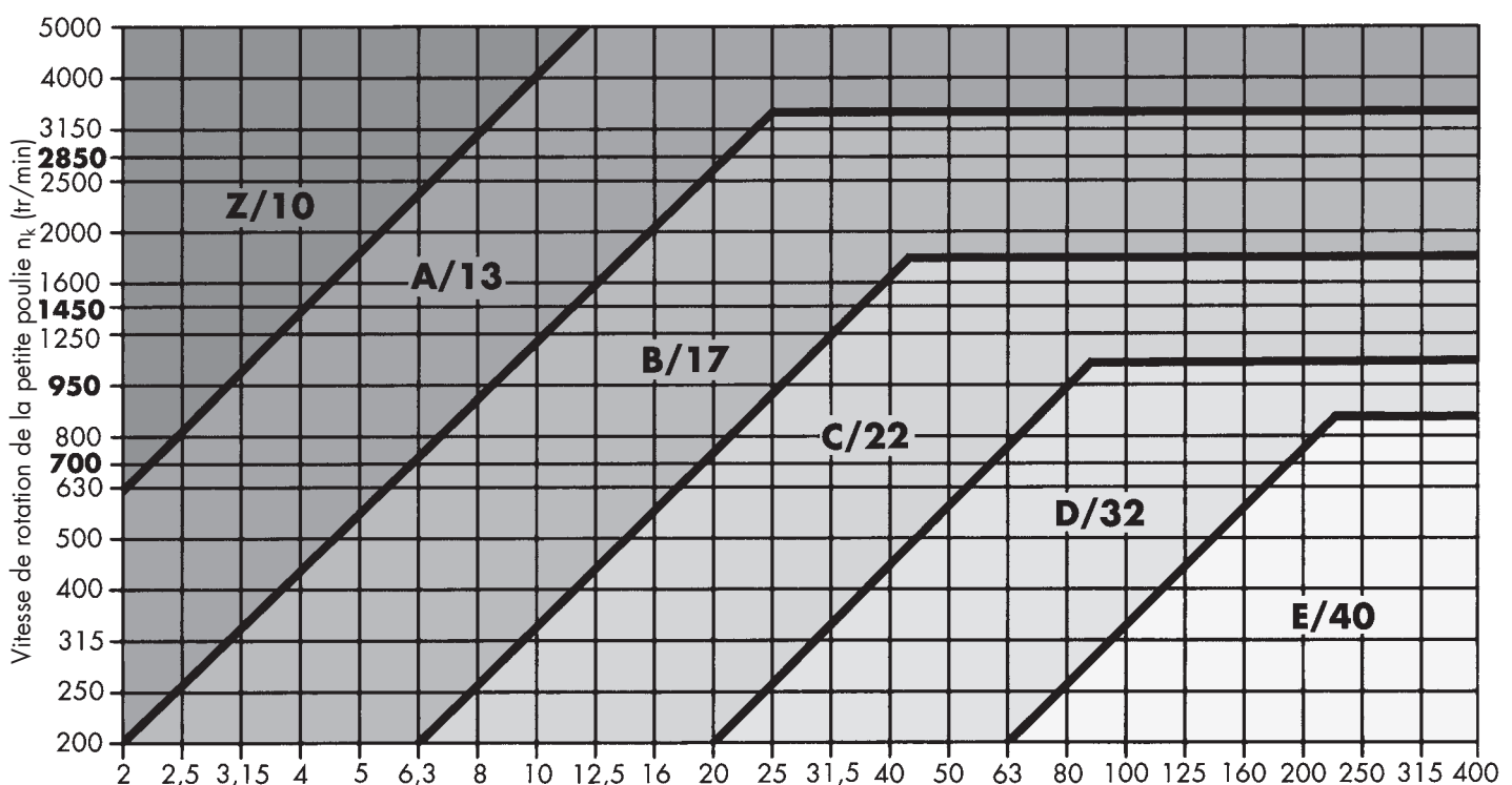
Diagramme 1: Optibelt VB courroies trapézoïdales classiques DIN 2215
