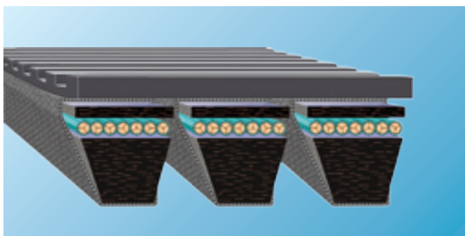
Courroie jumelée avec revêtement PKR 1
