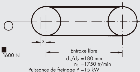
Banc d'essai - augmentation de l'entraxe [mm]
