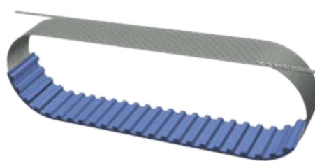
Structure de la courroie dentée optibelt ALPHA FLEX avec câble de traction S+Z enroulé hélicoïdalement et polyuréthane formé extrudé
