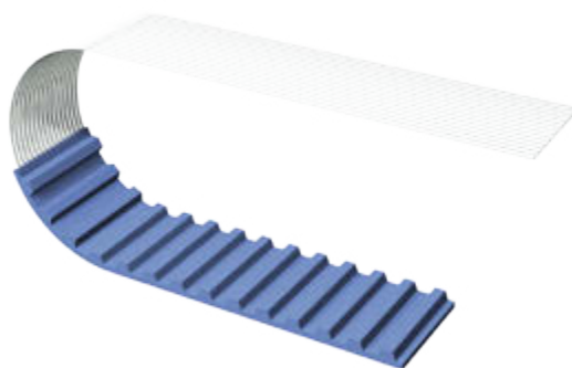
Structure de la courroie dentée optibelt ALPHA LINEAR avec câble de traction parallèle aux bords et polyuréthane extrudé, moulé
