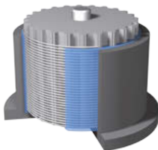
Procédé de fabrication par moulage pour courroies dentées optibelt ALPHA POWER, optibelt ALPHA TORQUE
