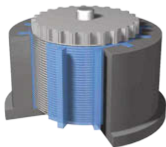
optibelt ALPHA SRP courroies dentées avec tasseaux
